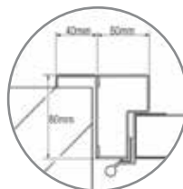
Frame afmetingen
