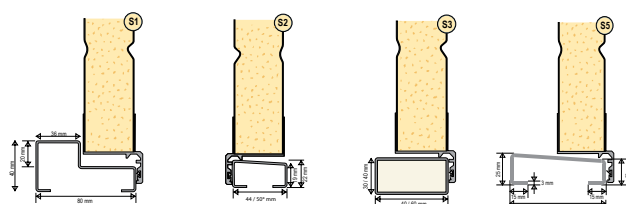
Frame met aanslagprofiel
